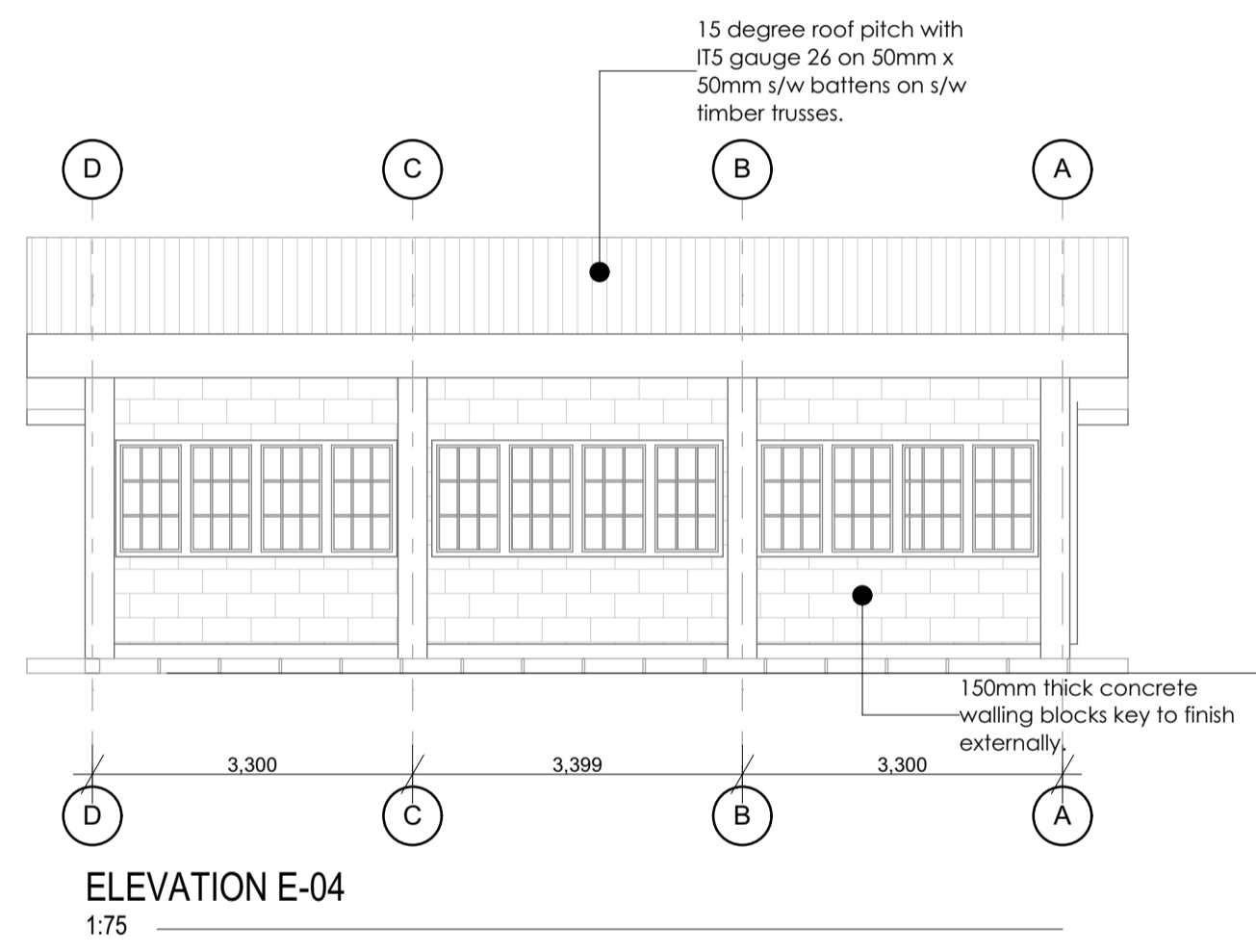
ELEVATION E-02 1:75
