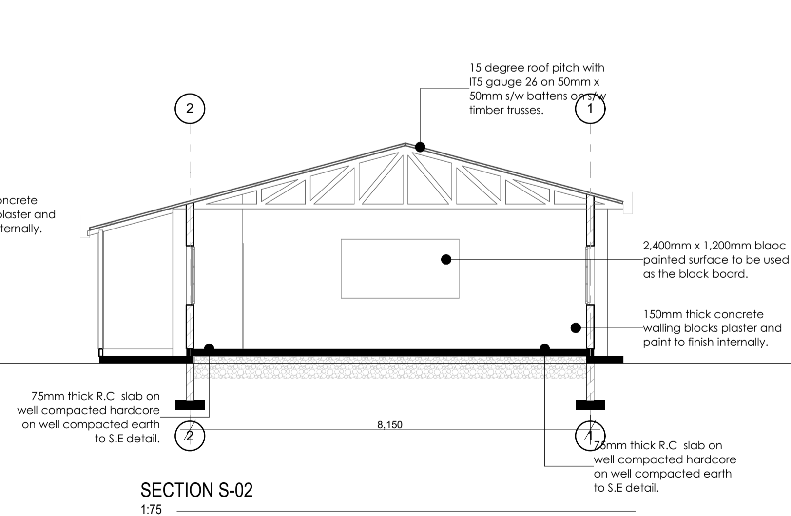
ELEVATION E-05 1:75
