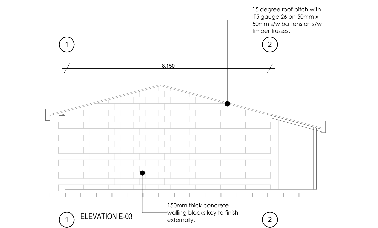
ELEVATION E-03 1:75
