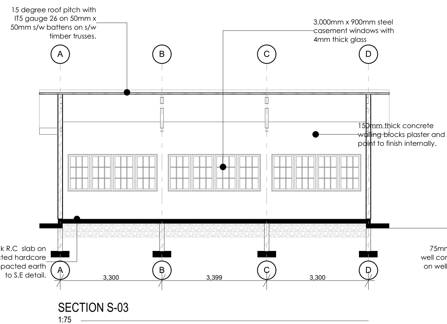
ELEVATION E-04 1:75
